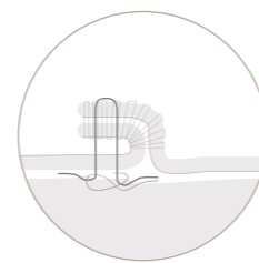
Seitennähte
